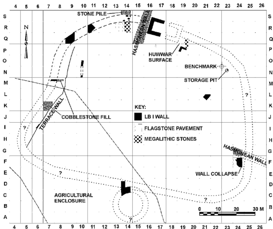
Рис. 3. Схема крепости периода поздней бронзы I в Хирбет эль-Макатире 22
